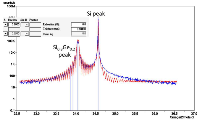
成長於Si(100)晶圓上的100nm厚度 \text{Si}_{0.8}\text{Ge}_{0.2} 單晶薄膜之XRD繞射曲線
