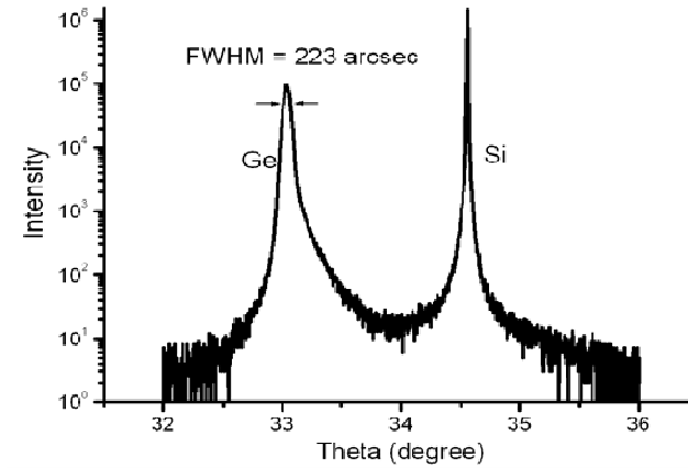
成長於Si(100)晶圓上的1.0 \mu\text{m} 厚度 Ge單晶薄膜之XRD繞射曲線
